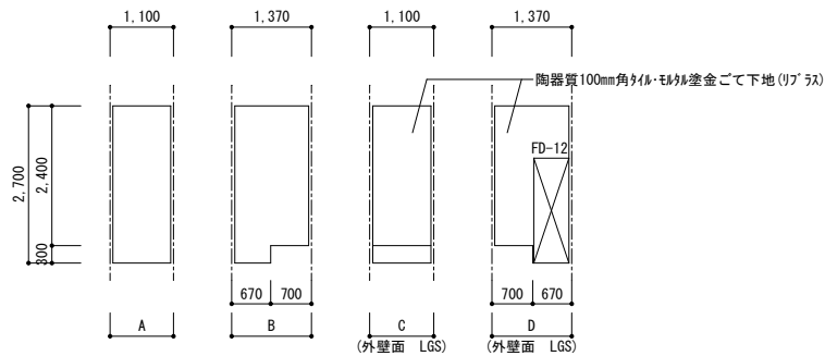
10:便所 特記なき仕上げは 陶器質100mm角タイル(CB)
