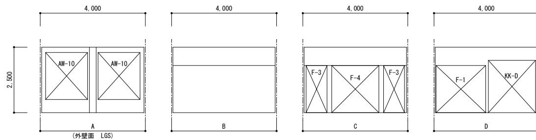
18:和室8帖 特記なき仕上げは ビニル材張:PB下地(LGS)、畳寄せ、付け鴨居
