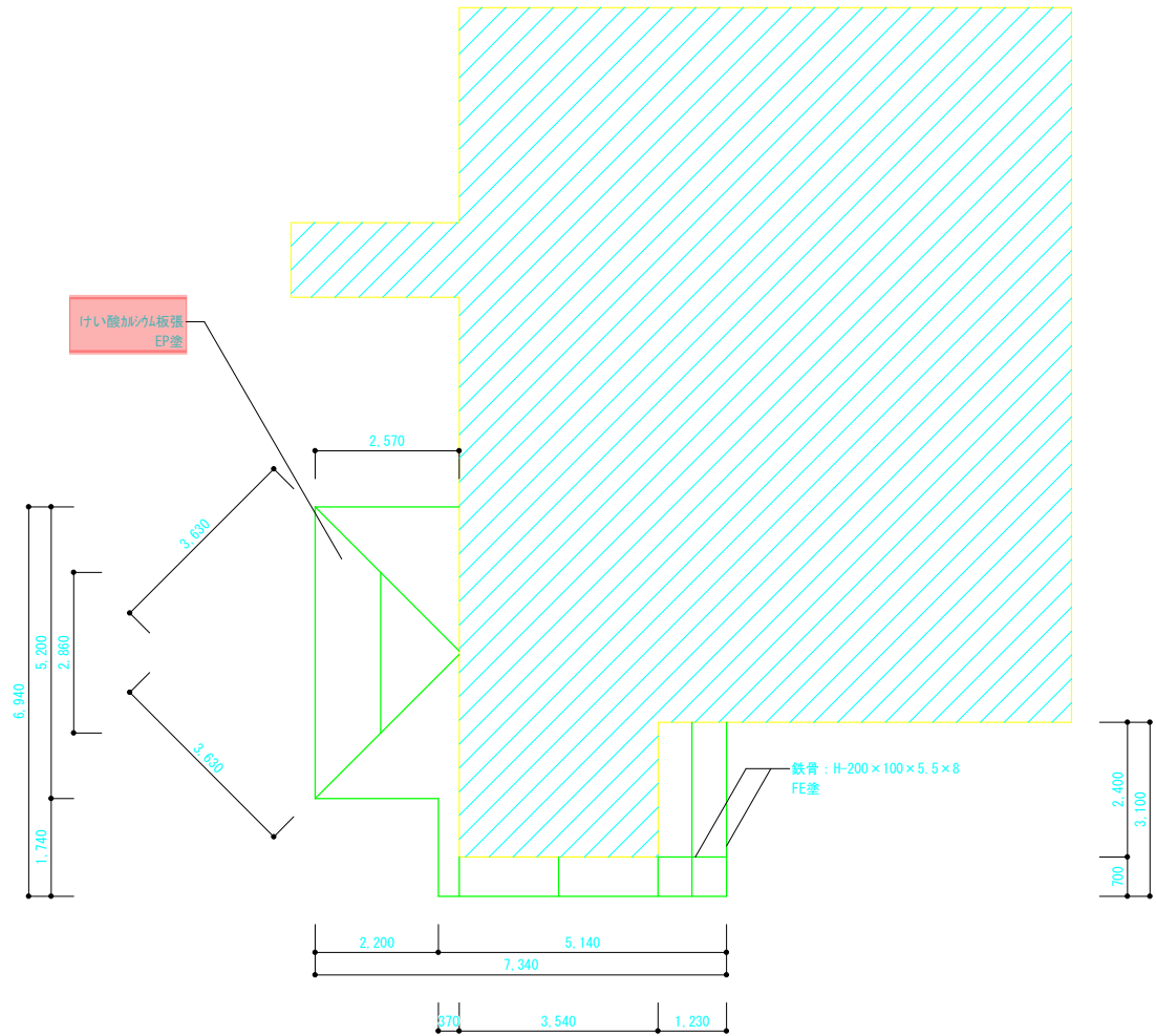
1 階軒天井伏図 S=1/150
