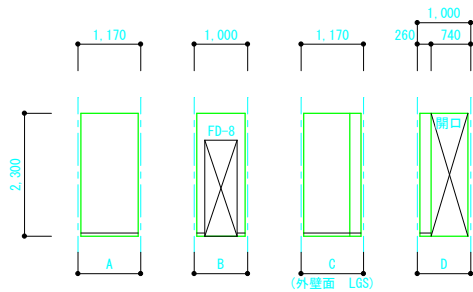
15:路込 特記なき仕上は ビニル紙張:PB下地(LGS)、木製幅木OS塗
