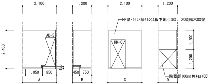
36: 手洗所 特記なき仕上りは EP 塗・セラミ塗金ごて下地 (CB)、木製幅木 OS 塗
