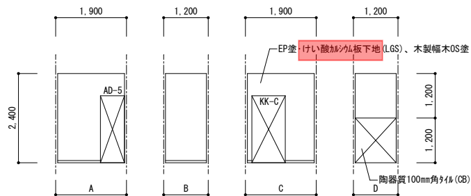
12:手洗所 特記なき仕上げは EP塗・モルタル塗金こて下地(CB)、木製幅木OS塗
