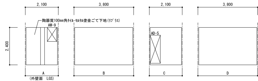
17:踏込 特記なき仕上げは ビニル材張:PB下地(LGS)、木製幅木OS塗
