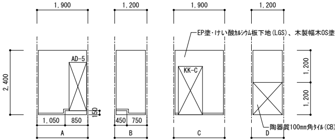
35: 手洗所 特記なき仕上りは EP 塗・セラミ塗金ごて下地 (CB)、木製幅木 OS 塗
