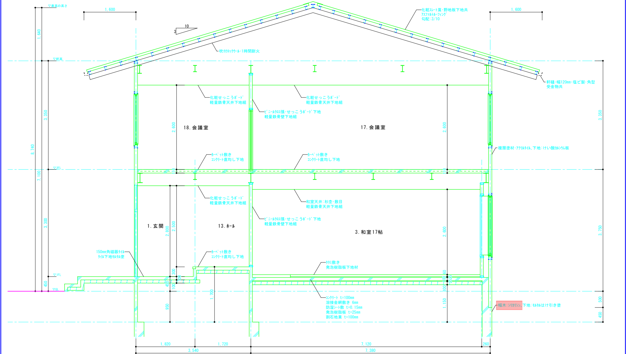
矩 計 図 S=1/50
