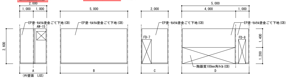
34: 洗面所 特記なき仕上りは EP 塗・けい酸ガラス板下地 (LGS)、木製幅木 OS 塗
