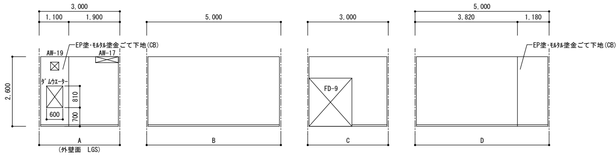
33: 配膳室 特記なき仕上りは EP 塗・けい酸ガラス板下地 (LGS)、木製幅木 OS 塗
