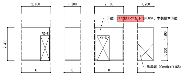
13:手洗所 特記なき仕上げは EP塗・モルタル塗金こて下地(CB)、木製幅木OS塗
