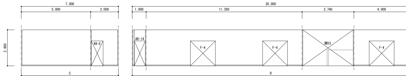
41. 廊下 特記なき仕上げはビニル貼張:PB下地(LGS)、木製幅木OS塗
