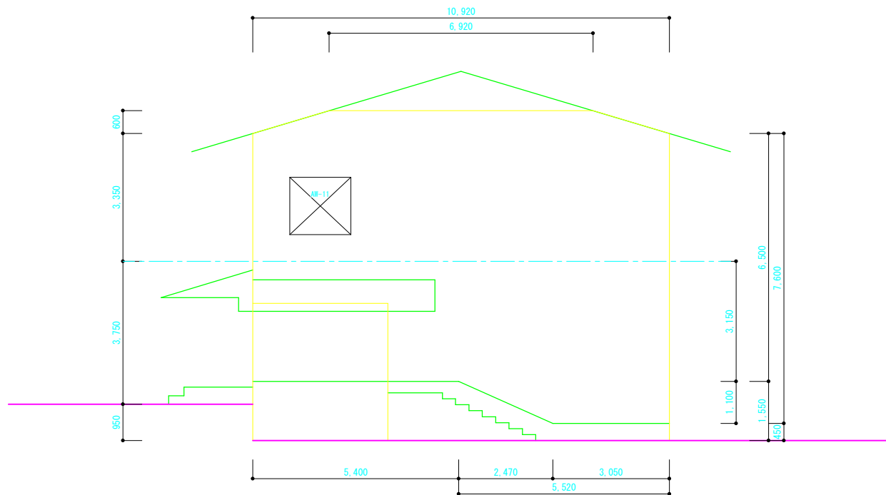
渡り廊下西立面図
