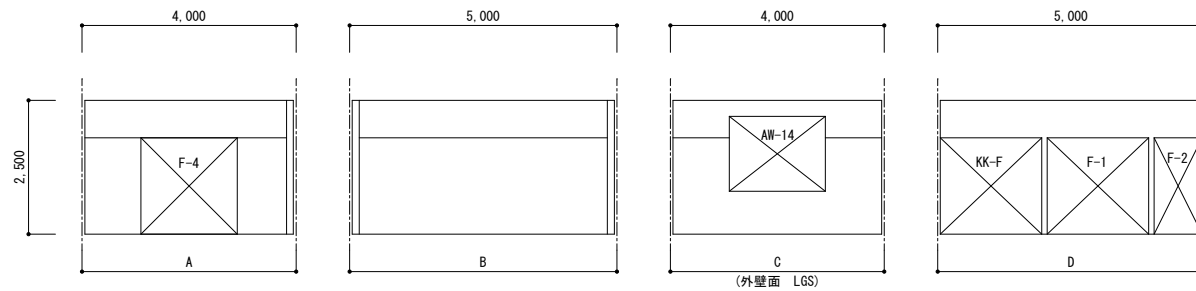
43. 和室10帖 特記なき仕上げはビニル貼張:PB下地(LGS)、畳寄せ、付け鴨居
